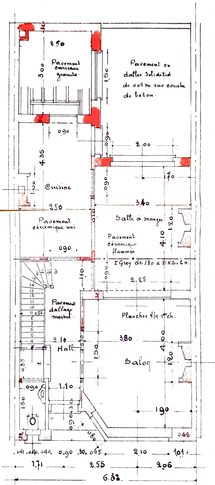
REZ-DE. CHAUSSEE.
