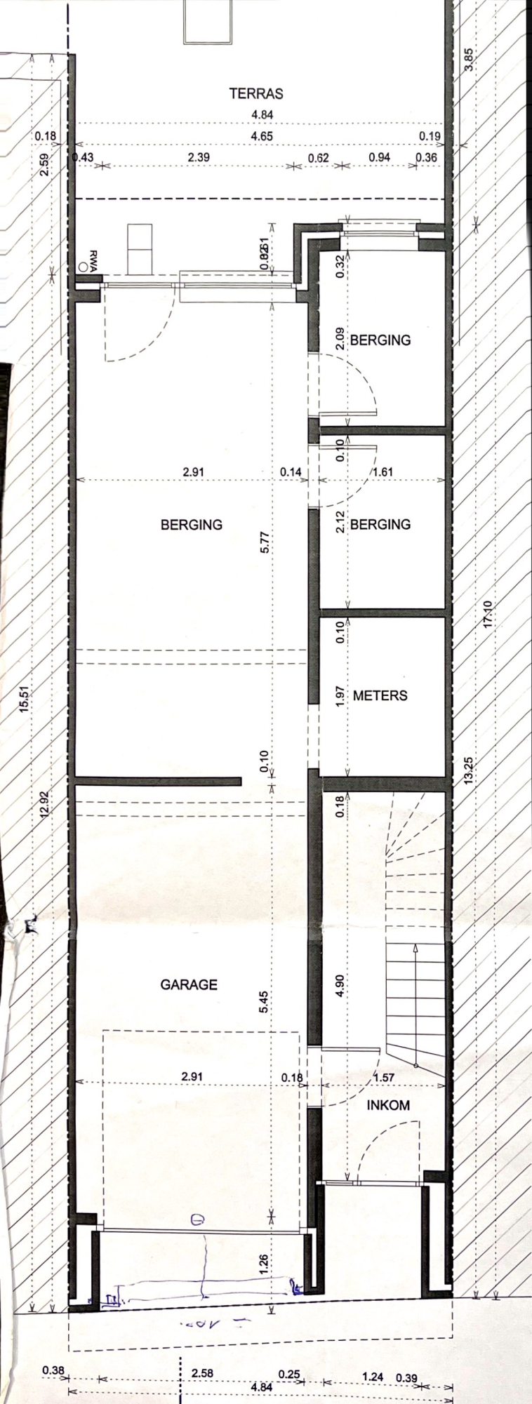
gelijkvloers | schaal 1/50
